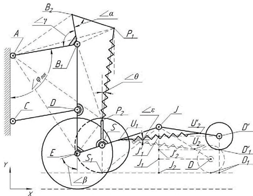
Рисунок 1 – Схематична модель дослідження зміни геометричних розмірів під час експлуатації посівної секції в режимі «максимум» Агро-Союз Turbosesem II 19-60 Джерело: [6]
