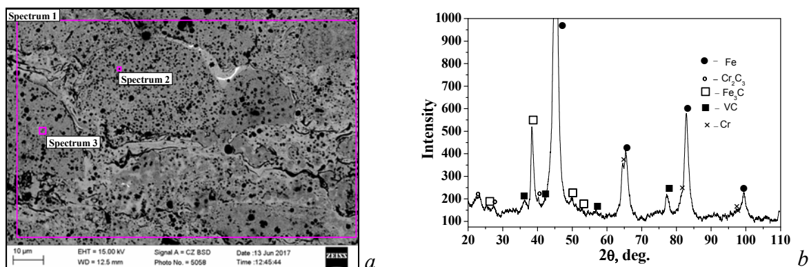
Рисунок 1 – Мікроструктура (а) та фазовий склад (б) HVOF покриття FeCr-VC
